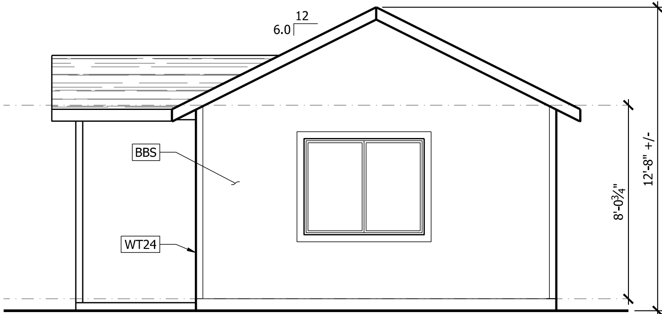
C RIGHT ELEVATION
